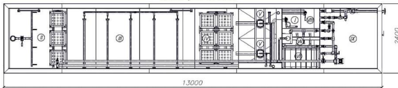
План установки
