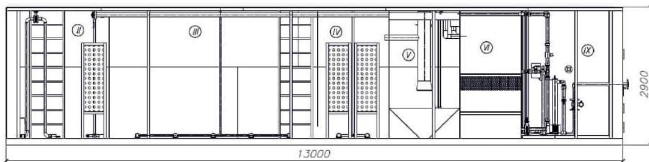
План установки
